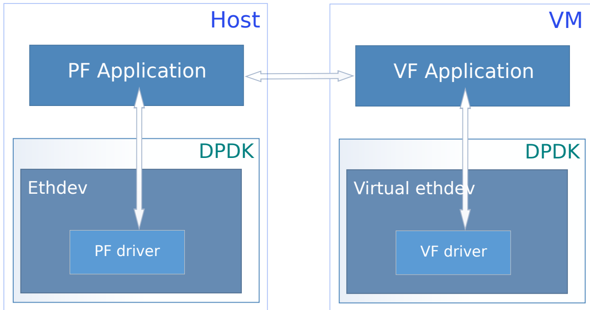
Fig. 5.1: VF daemon (VFd) Overview
