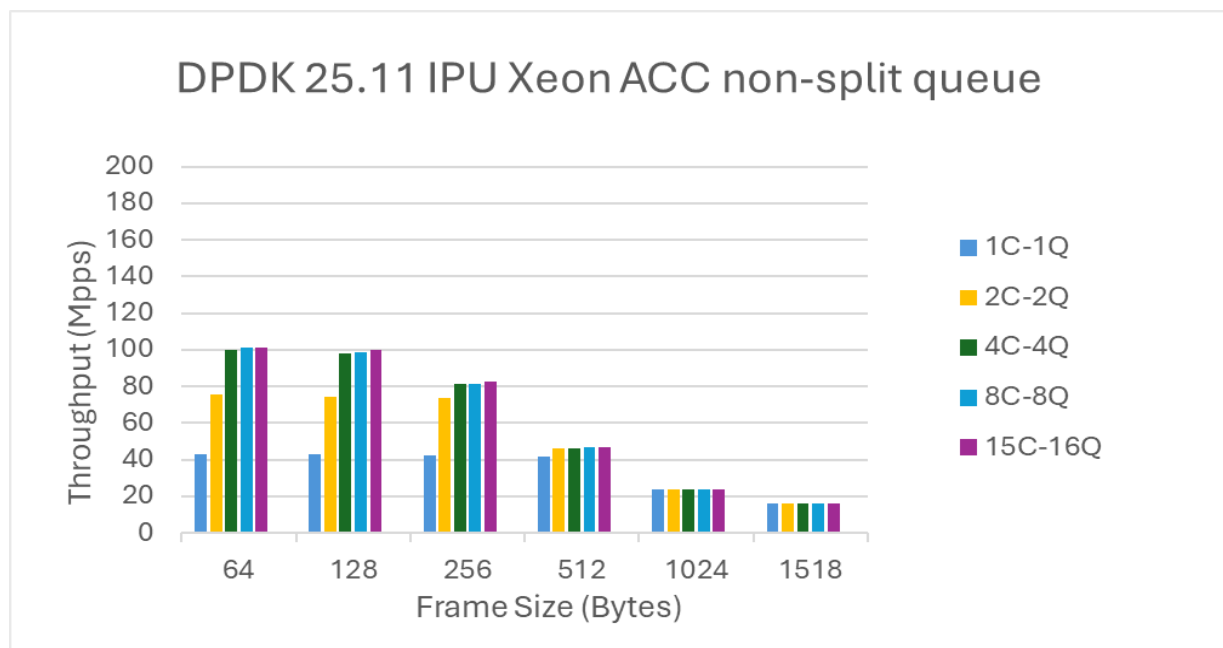
Figure 30: non-split queue on 1x Intel® IPU Adapter E2100-CCQDA2
