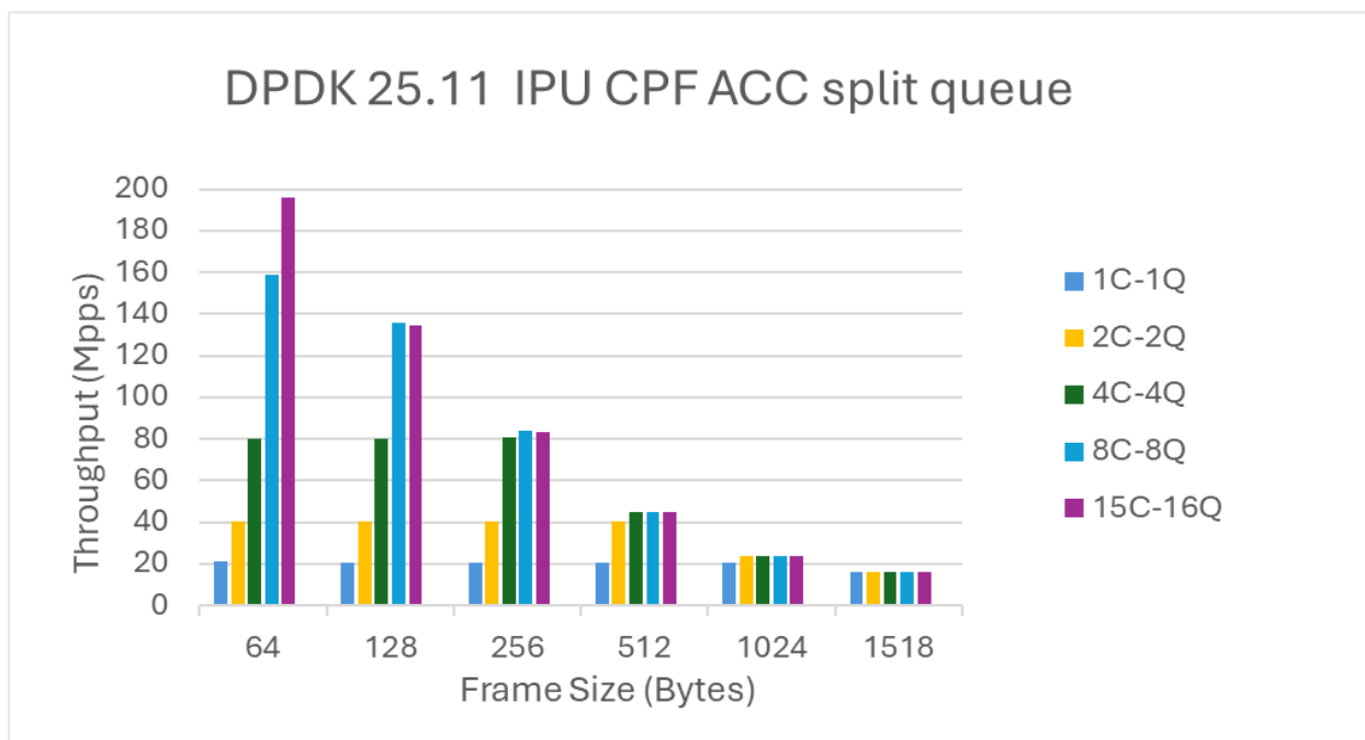
Figure 26: ACC split queue on 1x Intel® IPU Adapter E2100-CCQDA2
