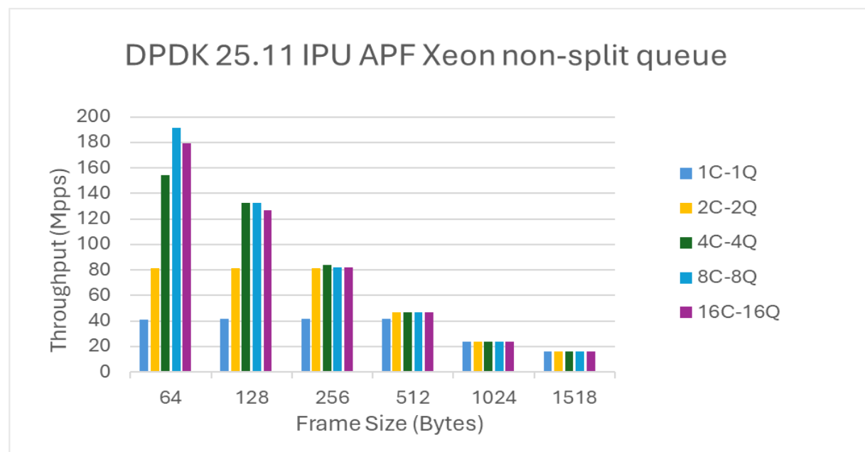
Figure 24: Xeon non-split queue on 1x Intel® IPU Adapter E2100-CCQDA2
